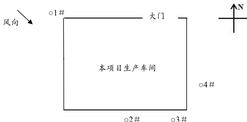
图 3-2 无组织废气检测点位图
