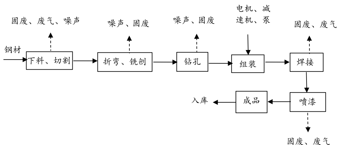
图 2-4 本项目生产工艺流程及产污环节图
