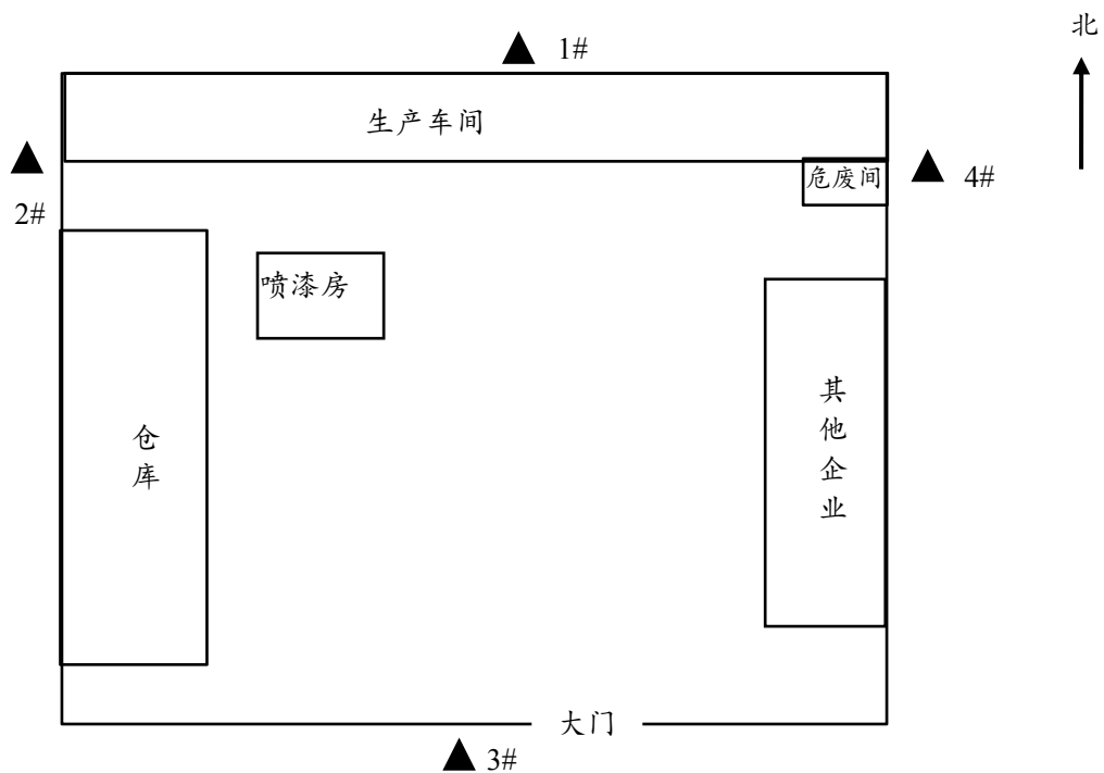
图 3-3 噪声检测点位图
