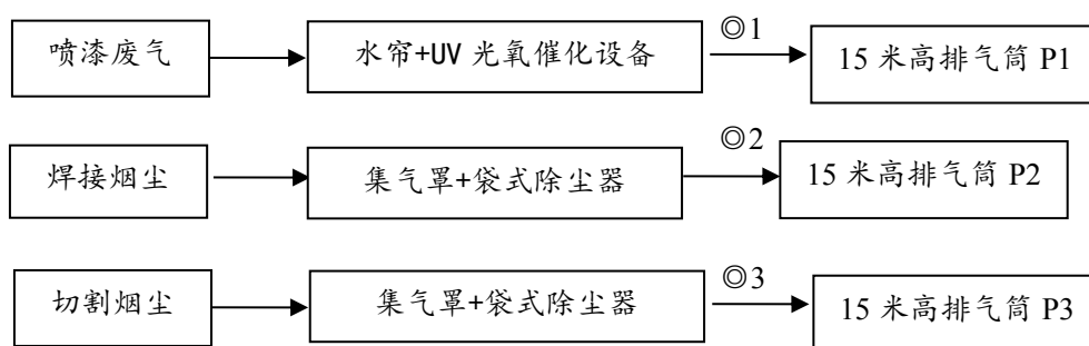
图 3-1 有组织废气监测点位
