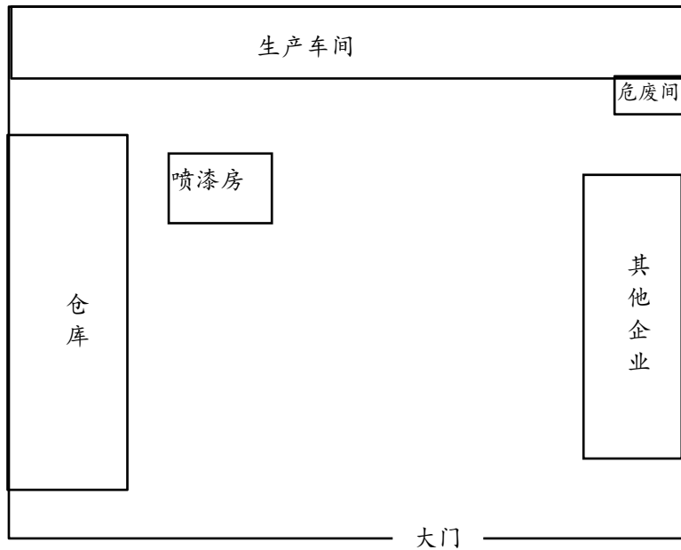
图 2-2 平面布置图
