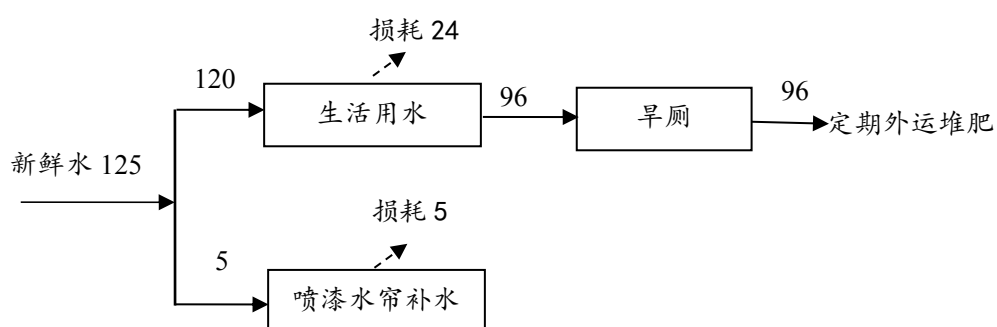
图 2-3 本项目水平衡图
