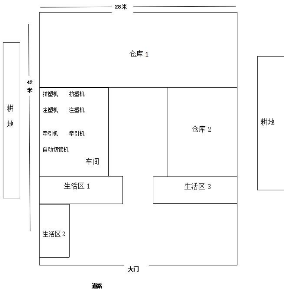
图 2-2 平面布置图
