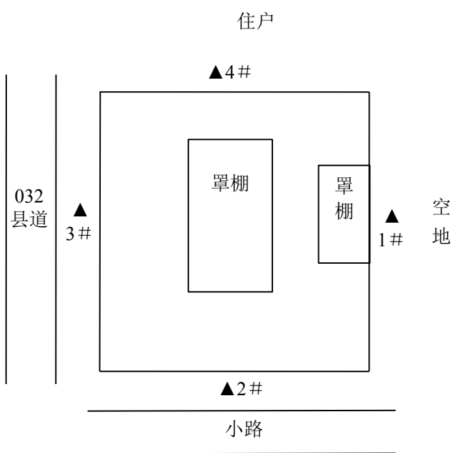
图 3-2 噪声检测点位图
