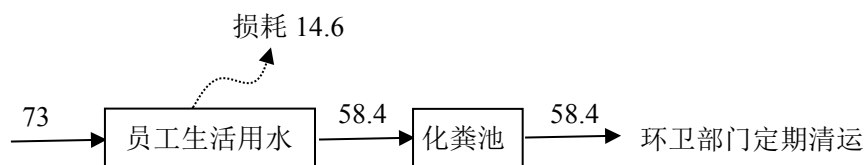
图 2-3 项目水平衡图 (m³/a)
