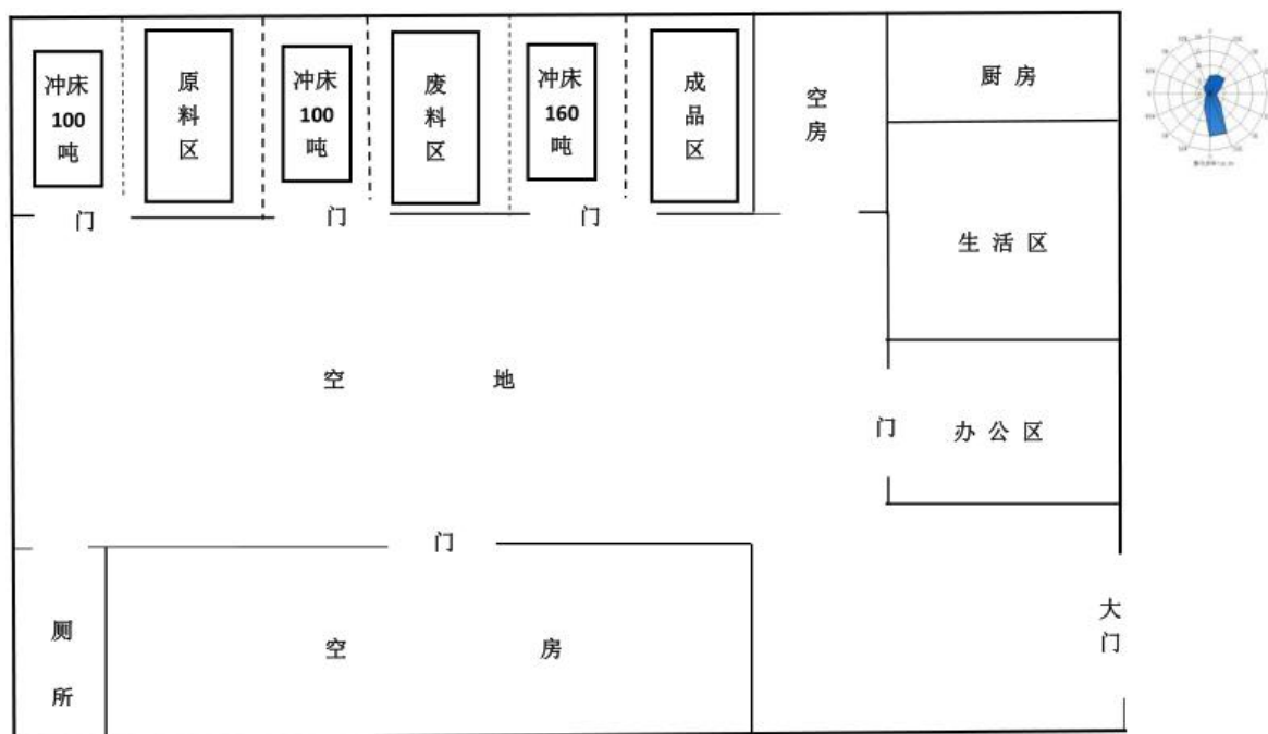
图 2-2 平面布置图
